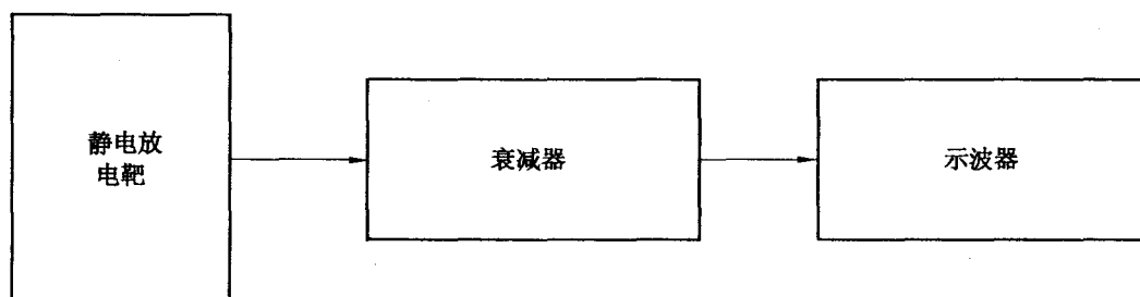
图 5 连接示意图
