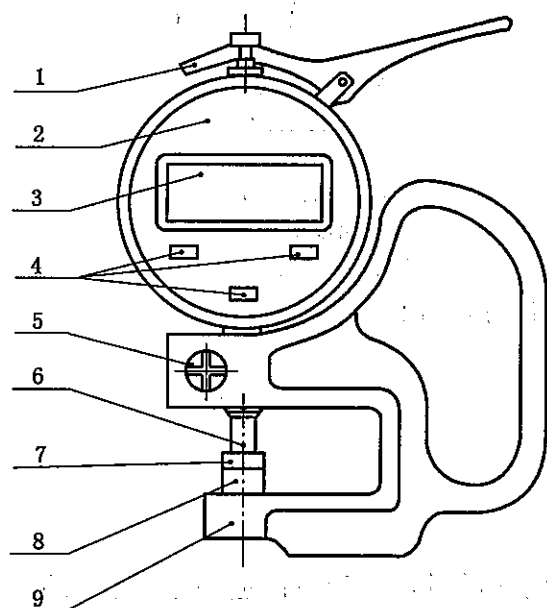
(a) 数显式厚度表
