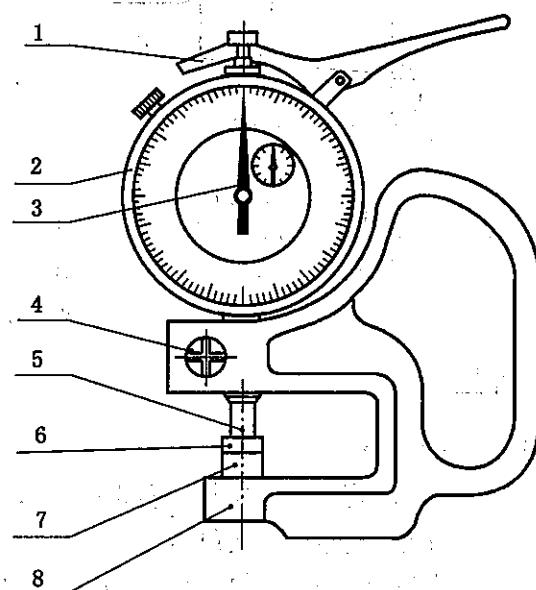
(b) 指针式厚度表
